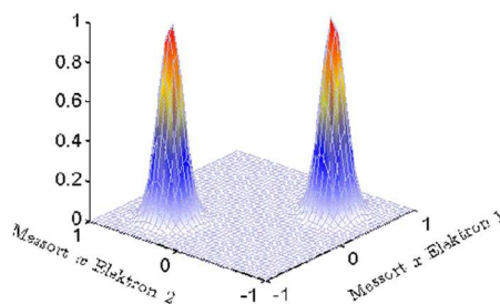
Abbildung 7-3 Quantenmechanische Wahrscheinlichkeit dafür, Elektron 1 an dem an der rechte Koordinaten angegebenen Ort zu messen und Elektron 2 an dem an der linken Koordinaten. Beide Koordinaten beschreiben auf derselben x-Achse! Die Verteilung ist wegen der Ununterscheidbarkeit der Elektronen symmetrisch. Beide Fälle sind gleich Wahrscheinlich: Elektron 1 um x=0.5 und Elektron 2 um x=-0.5 oder Elektron 1 um x=-0.5 und Elektron 2 um x=0.5 .
