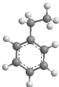
Ethylbenzene
