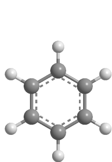
Benzene
