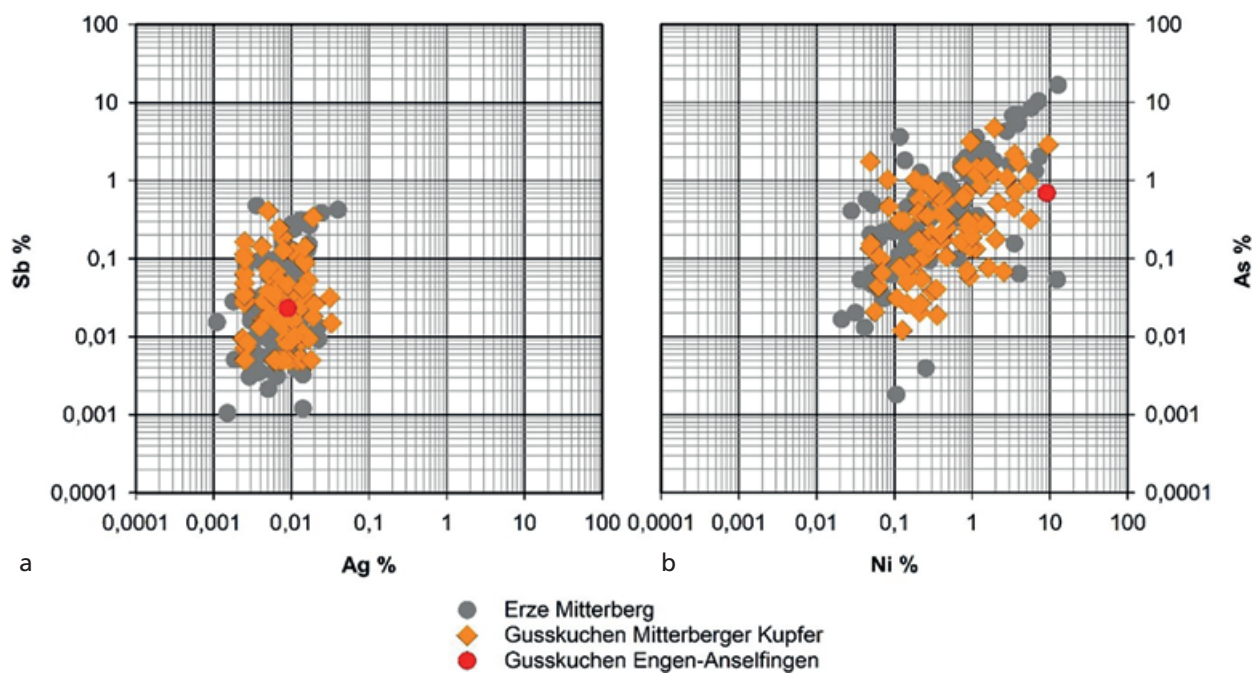
Abb. 7 Konzentrationen von Silber und Antimon (a) und Nickel und Arsen (b) in Erzen aus dem Mitterberger Revier und Gusskuchen aus Mitterberger Kupfer im Vergleich mit dem Gusskuchen von Anseltigen. – (Grafik J. Lutz).
